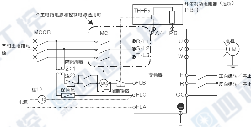
b) 使用没有温度保险丝的制动电阻器时
