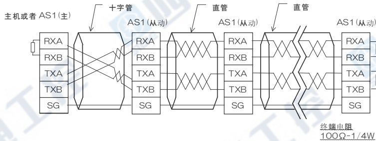
■配线时的注意事项
