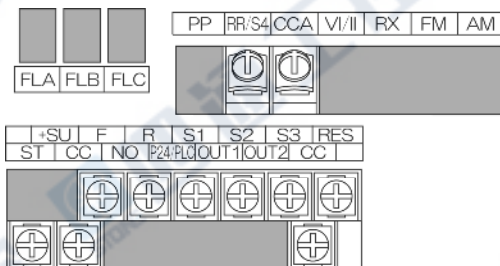
■接点输入端子的功能设定
