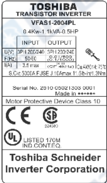
额定铭牌
