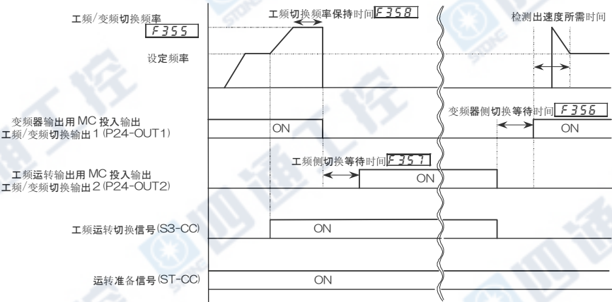
〔时间图表（设定示例）〕
