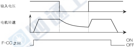
1）瞬停后再起动（瞬停再起动功能）
