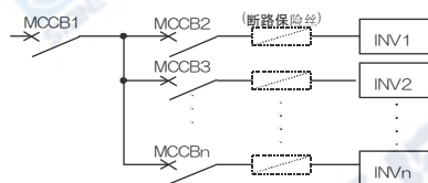
变频器的选择断路
