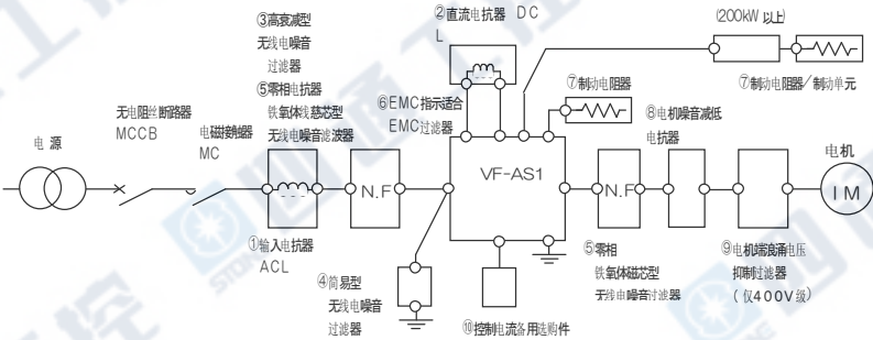
外置式选配件的种类
